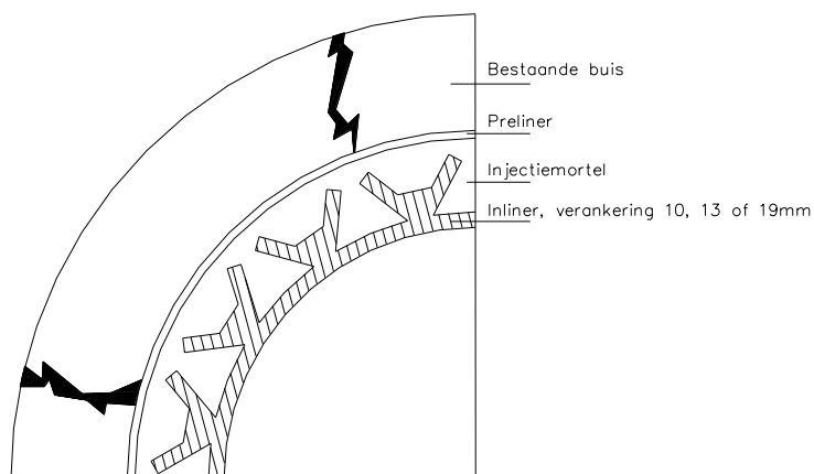
Figuur 7-23-1: opbouw systeem
