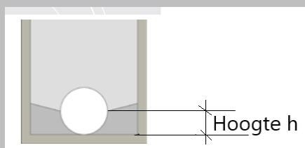
Figuur 7-3-A: minimale hoogte banket bij ronde en vierkante put
