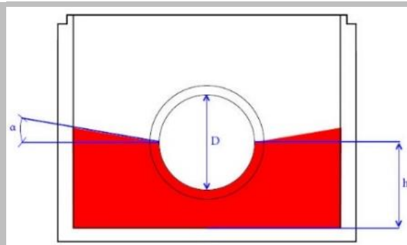
Figuur 7-3-B: hoek \alpha van het banket
