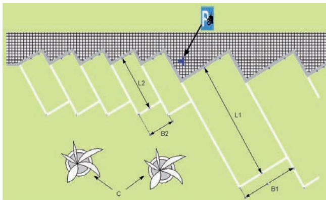
Parkeerplaats schuin tegenover de rijbaan
