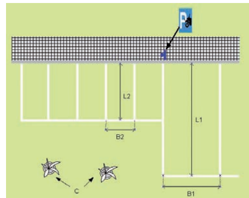
Parkeerplaats haaks op de rijbaan
