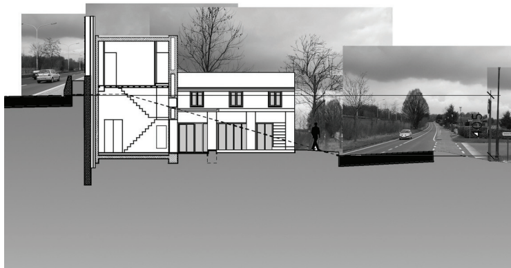
Snede door scherm en woning
