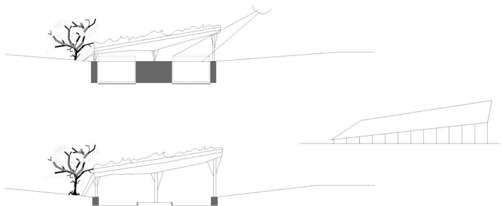
Doorsnedes
